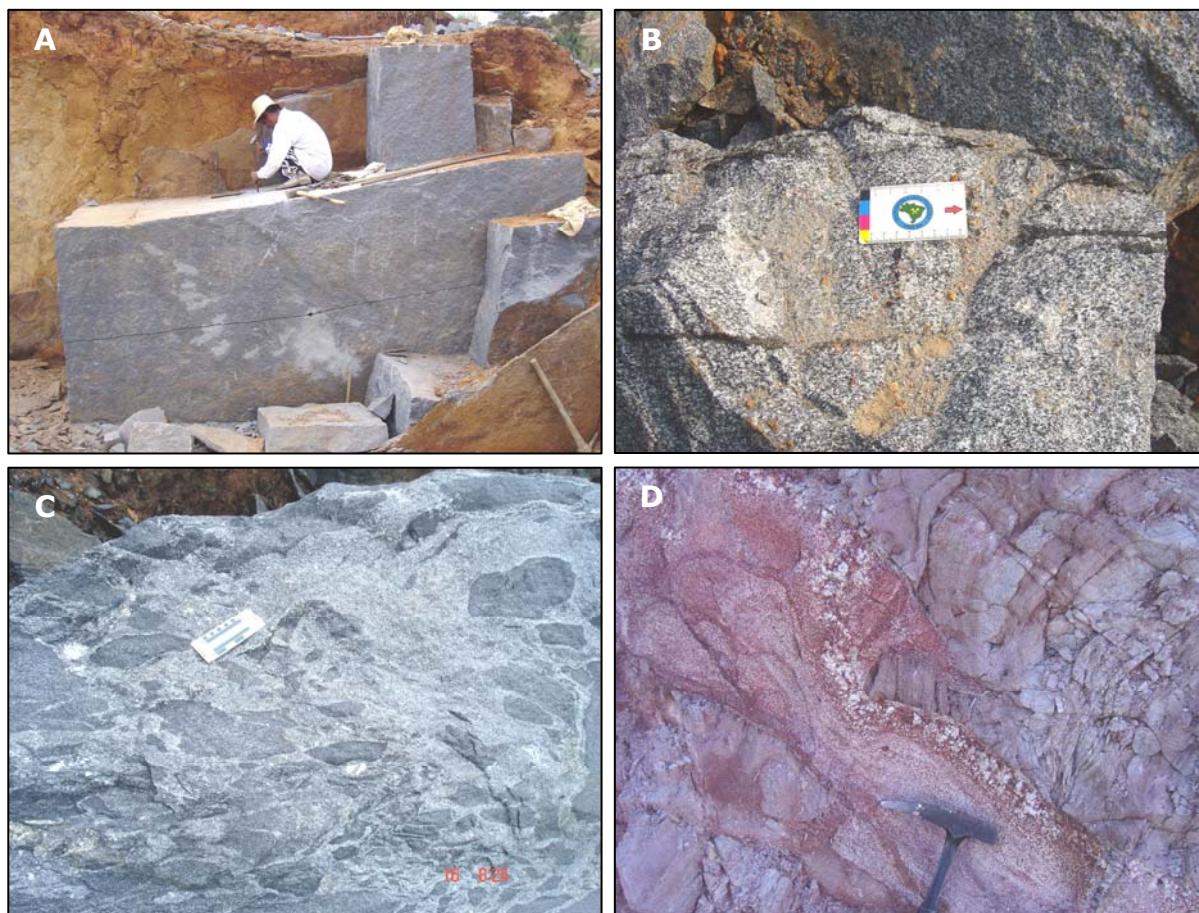
Figura 20: Biotita-hornblenda gnaiss. a) granulação fina e aspecto homogêneo são característicos (estação CN-198; 794686E/7760499N); b) foliação gnáissica bem desenvolvida (estação CN-198); c) enclaves quartzo-dioríticos indicando processo de magma mingling (estação CN-341; 808139E/ 7755460N); d) contato intrusivo com quartzito Andrelândia (estação CN-137; 792961E/7780956N).
