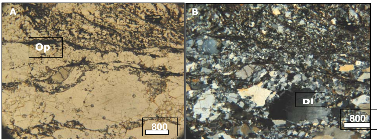
Figura 11: Gnaiss enderbítico do Complexo Juiz de Fora, exibindo textura milonítica com evidências de recristalização dinâmica e individualização de subgrãos dos enderbitos (amostra CN20;800918E/7737407N). a) nicóis paralelos; b) nicóis cruzados.
