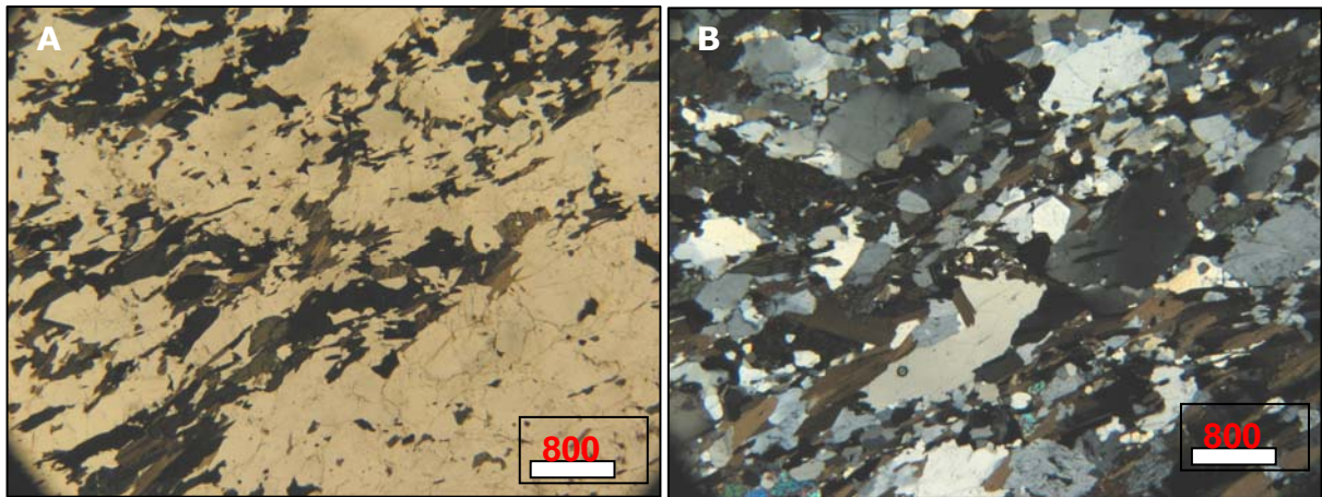
Figura 7: Associação mineral típica dos gnaisses do Complexo Mantiqueira (quartzo + plagioclásio + biotita + anfibólio; amostra CN 218; 763712E/7772997N). a) nicóis paralelos; b) nicóis cruzados.
