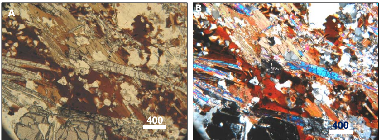
Figura 14: Grupo Andrelândia, feições microscópicas do paragnaisse. a) sillimanita-biotita granada gnaisse, nicóis paralelos (amostra CN 420; 804930E/7781862N); b) idem anterior, nicóis cruzados.
