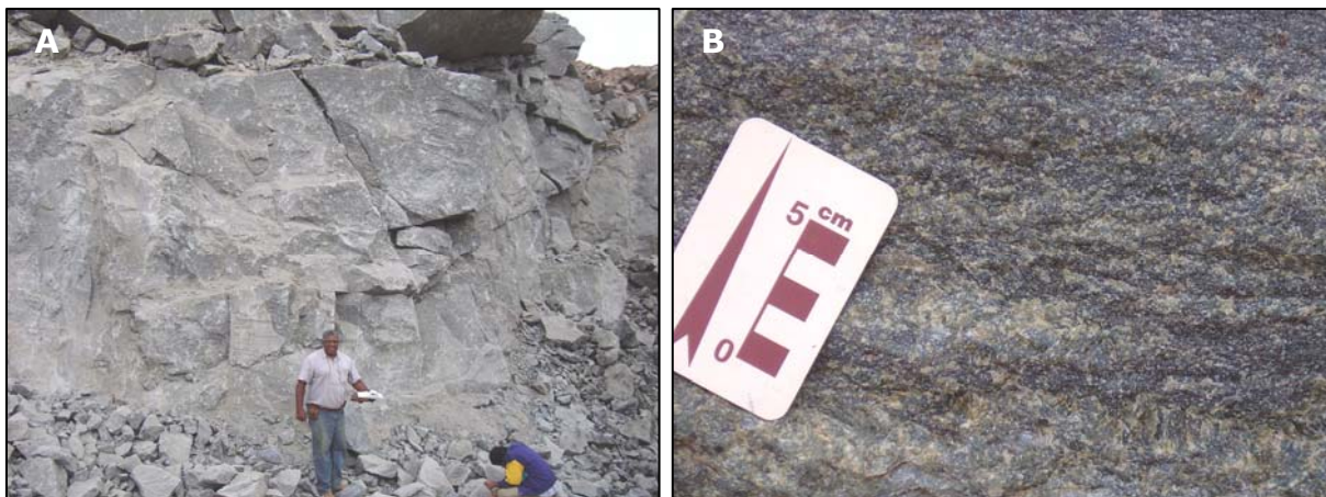
Figura 21: Charno-enderbitos. a) vista geral de afloramento, mostrando o aspecto homogêneo da rocha (estação CN-198; 794686E/7760499N); b) detalhe de charno-enderbitito, granulação média, com granada.
