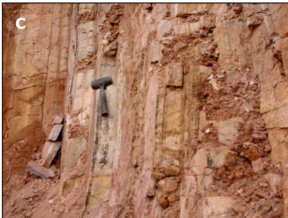
Figura 18: Grupo Andrelândia, quartzito. a) camada espessa de quartzito puro, aspecto estratificado (estação CN-148; 790704E/7765364N); b) contato transicional entre quartzito e paragneisse sapolitizado (estação CN-156; 791556E/7773520N); c) alternância de leitos de quartzito e paragneisse (estação CN-156).
