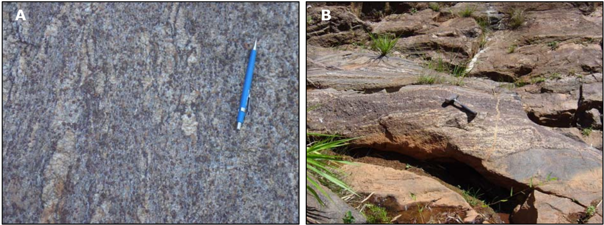
Figura 15: Grupo Andrelândia, feições macroscópicas do paragneisse. a) porção rica em granada, com mobilizados leucocráticos em vênulas (estação CN-206; 770288E/7774449N); b) leito com alta concentração de granada (estação CN-213; 772618N/7784754N).
