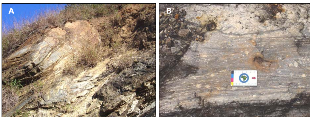
Figura 26: Estruturas mesoscópicas nas grandes zonas de cisalhamento. a) Zona de Cisalhamento de Abre Campo, gnaisse Mantiqueira no contato com paragneisse Andrelândia (estação CN-209; 767973E/7775697N); b) milonito de biotita-hornblenda gnaisse no domínio da Zona de Cisalhamento de Manhuaçu (estação CN-356; 795316E/7774406N).
