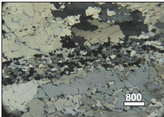
Figura 19: Aspecto do quartzito do Grupo Andrelândia em lâmina delgada, nicóis cruzados (amostra CN 281a; 794646E/7744648N).
