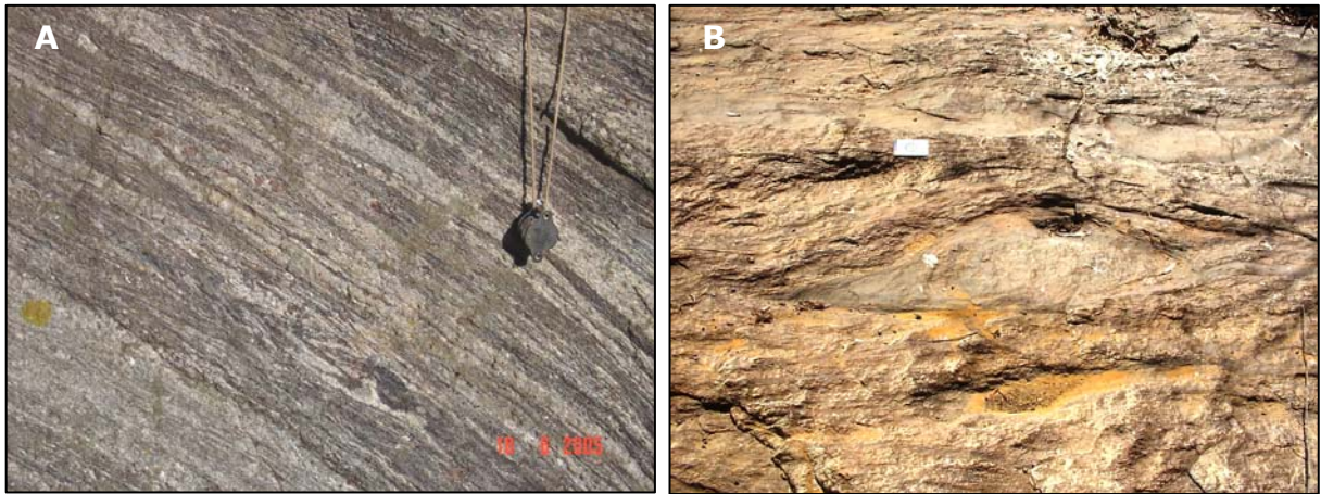
Figura 13: Grupo Andrelândia, feições macroscópicas do paragnaisse (biotita-granada gnaisse. a) bandamento fino característico, granada esparsa (estação CN-20; 800918E/7737407N); b) corpos tabulares, boudinados, de anfibólito no paragnaisse (estação CN-285; 791012E/7745465N).
