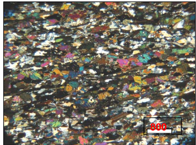
Figura 24: Aspecto microscópico de dique máfico; textura orientada e composição mineralógica apresentando hornblenda, clinopiroxênio, plagioclásio, biotita e quartzo (nicóis cruzados, amostra CN 345d; 809475/ 7755031N).
