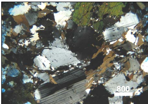
Figura 22: Aspecto microscópico do charno-enderbitito (amostra CN-114; 779503E/7750224N).
