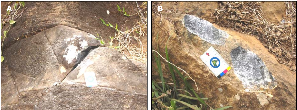
Figura 23: Corpos máficos. a) dique de anfibolito cortando paragneisse (Estação CN-248; 807132E/ 7752050N; b) bloco de metagabro (CN-246).
