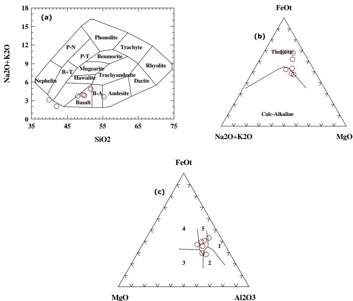
Figura 33: Diques máficos. a) Diagrama de classificação de rochas ígneas, de Cox et al. (1979); b) diagrama de Irvine & Baragar (1971); c) diagrama de Pearce et al. (1977); o campo 5 é dos basaltos continentais.
