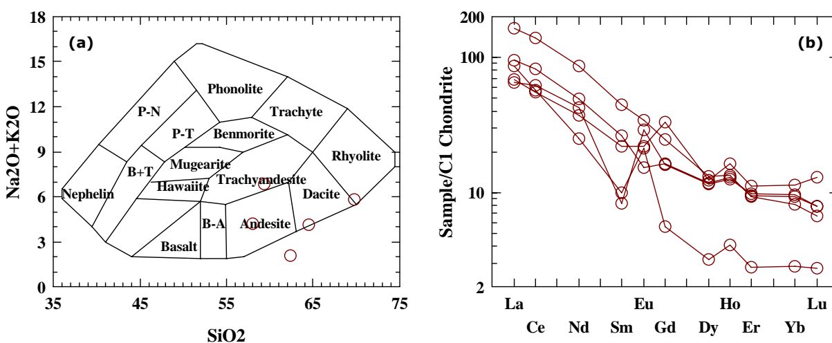
Figura 32: Gnaisses enderbíticos do Complexo Juiz de Fora. a) diagrama de classificação de rochas ígneas, de Cox et al. (1979); b) diagrama de ETR.
