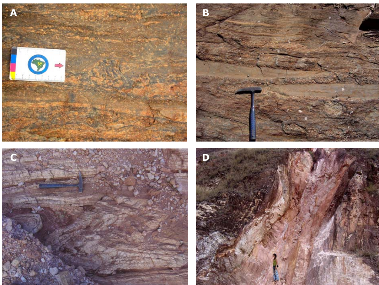
Figura 30: Estruturas no domínio da Zona de Cisalhamento de Manhuaçu: a) milonito de paragnaisse com porfiroclasto indicando movimentação destal (estação CN-324; 783865E/7742689N); b) corpo de anfibolito rompido, indicando movimentação destal (estação CN-285; 791012E/7745465N); c) dobra apertada em camada de quartzito com eixo subvertical (estação CN-148; 790704E/7765364N); d) quartzito exibindo estrutura em flor (estação CN-195; 788960E/7753313N).
