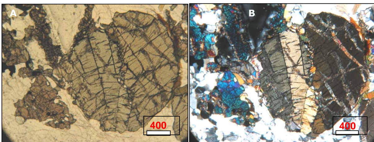
Figura 12: Detalhe de geminação mecânica em cristal de ortopiroxênio, gnaiss enderbítico (amostra CN 401;800780E/7783704N). a) nicóis paralelos; b) nicóis cruzados
