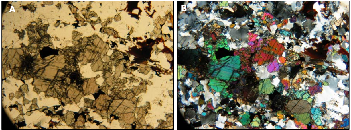
Figura 9: Textura granoblástica típica dos granulitos básicos da Complexo Juiz de Fora (amostra CN 2;766883E/7735650N). a) nicóis paralelos; b) nicóis cruzados
