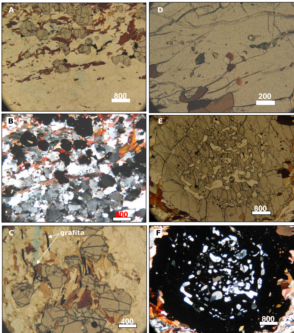
Figura 16: Grupo Andrelândia, feições microscópicas do paragnaisse, a) textura lepidoblástica típica do paragnaisse, nicóis paralelos (amostra CN 54; 766726E/7731832N); b) idem anterior, nicóis cruzados; c) detalhe de palhetas de grafita associadas à biotita, nicóis paralelos (amostra CN 54); d) inclusões de espinélio e biotita em cristal de granada, nicóis paralelos (amostra CN 27; 765018E/7747784N); e) inclusões de plagioclásio e quartzo em granada com estrutura snowball, nicóis paralelos (amostra CN 27); f) idem anterior, nicóis cruzados.
