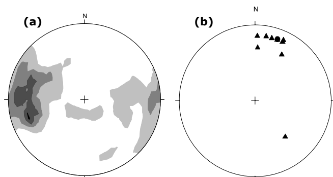
Figura 29: Elementos estruturais da porção E da área; a) Diagrama de contorno de polos da foliação principal (127 medidas, máximo em 71/76, contornos: 1, 3, 5, 7). B) Diagrama de elementos lineares (eixo de dobra ●, lineação mineral - ▲).
