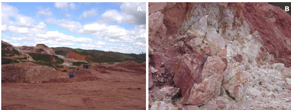
Figura 38: a) mina de caulim de Vermelho Novo (estação CN-140; 789328E/7778826E); b) detalhe de pegmatito na mesma mina.
