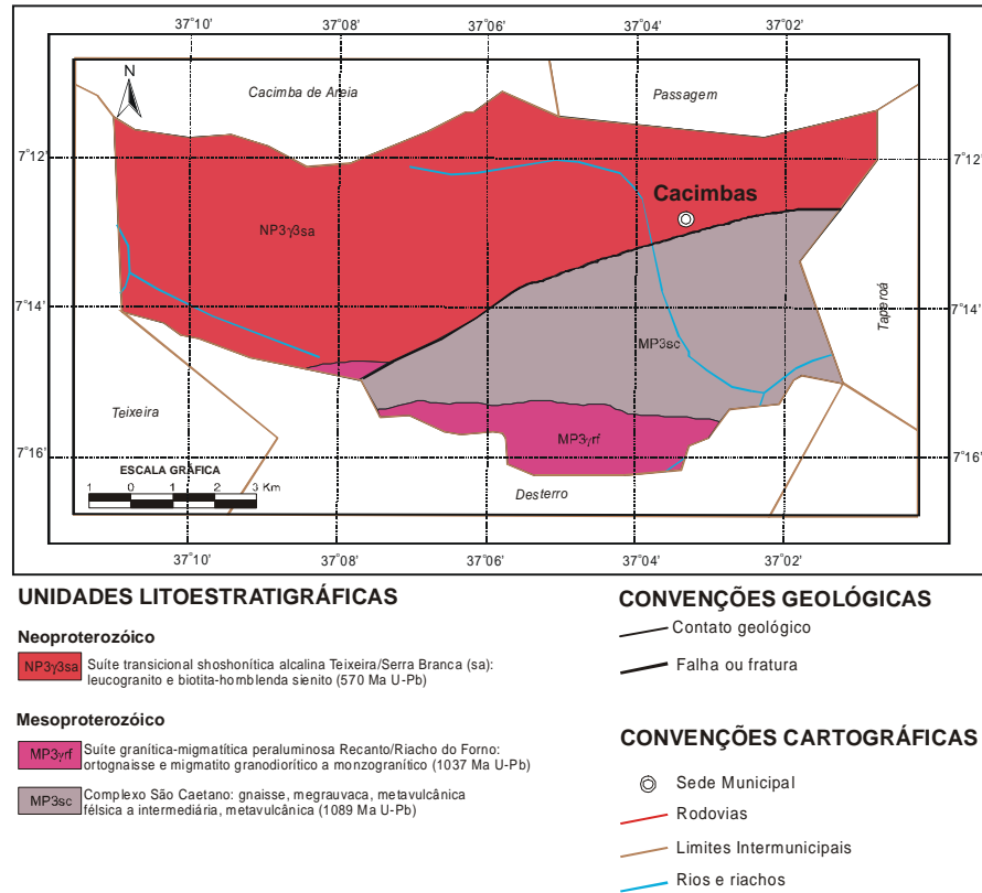
Figura 3 – Mapa Geológico
