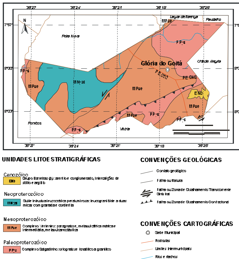
Figura 3 – Mapa Geológico
