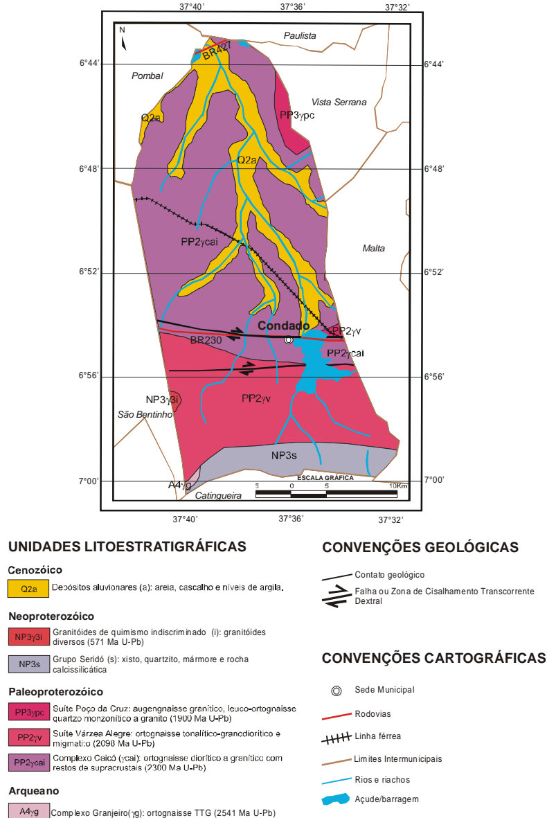
Figura 3 – Mapa Geológico
