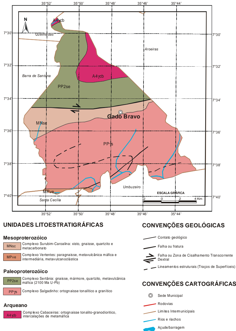
Figura 3 – Mapa Geológico
