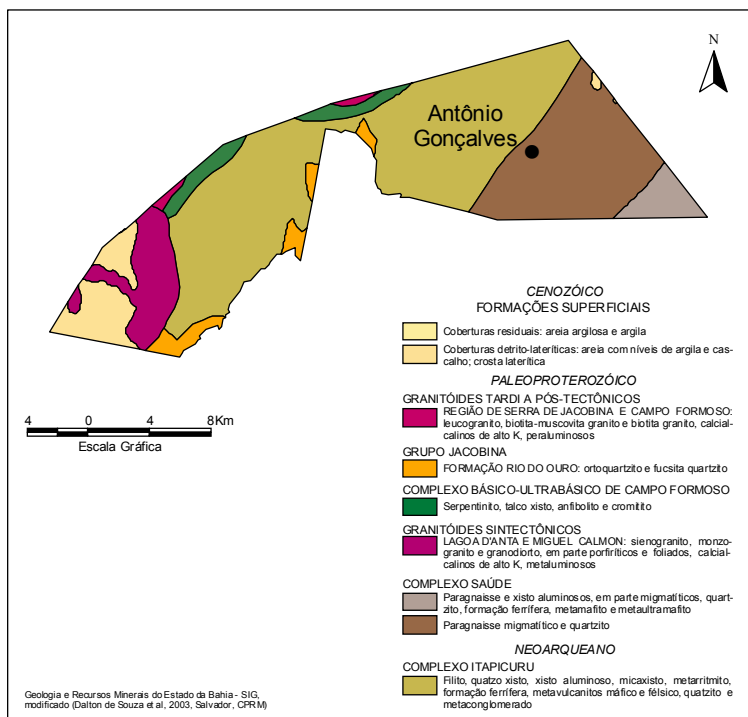
Figura 3 – Esboço geológico.
