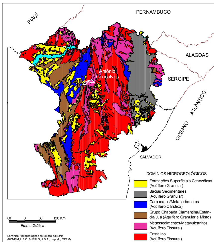
Figura 4 – Domínio hidrogeológico.
