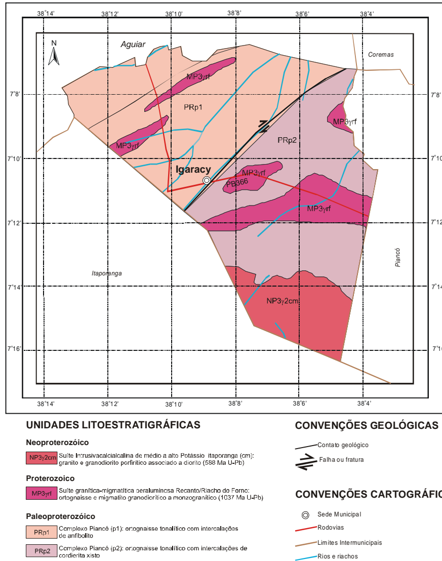
Figura 3 – Mapa Geológico
