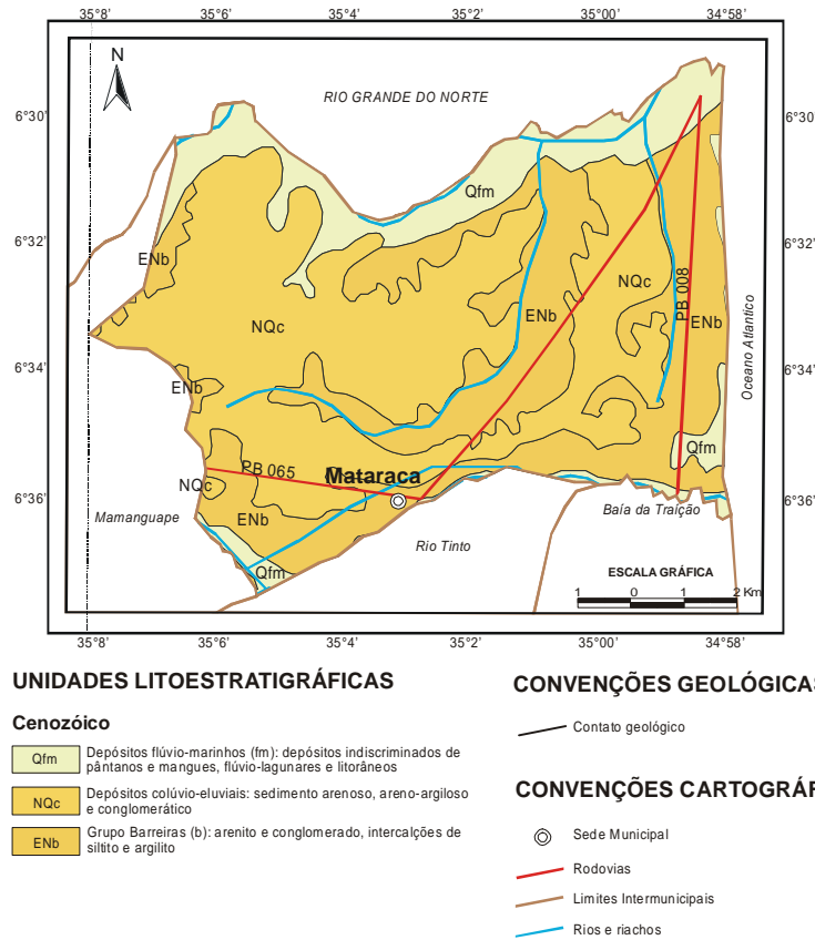
Figura 3 – Mapa Geológico
