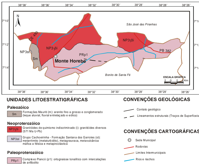
Figura 3 – Mapa Geológico
