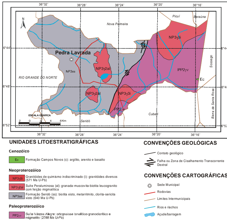
Figura 3 – Mapa Geológico
