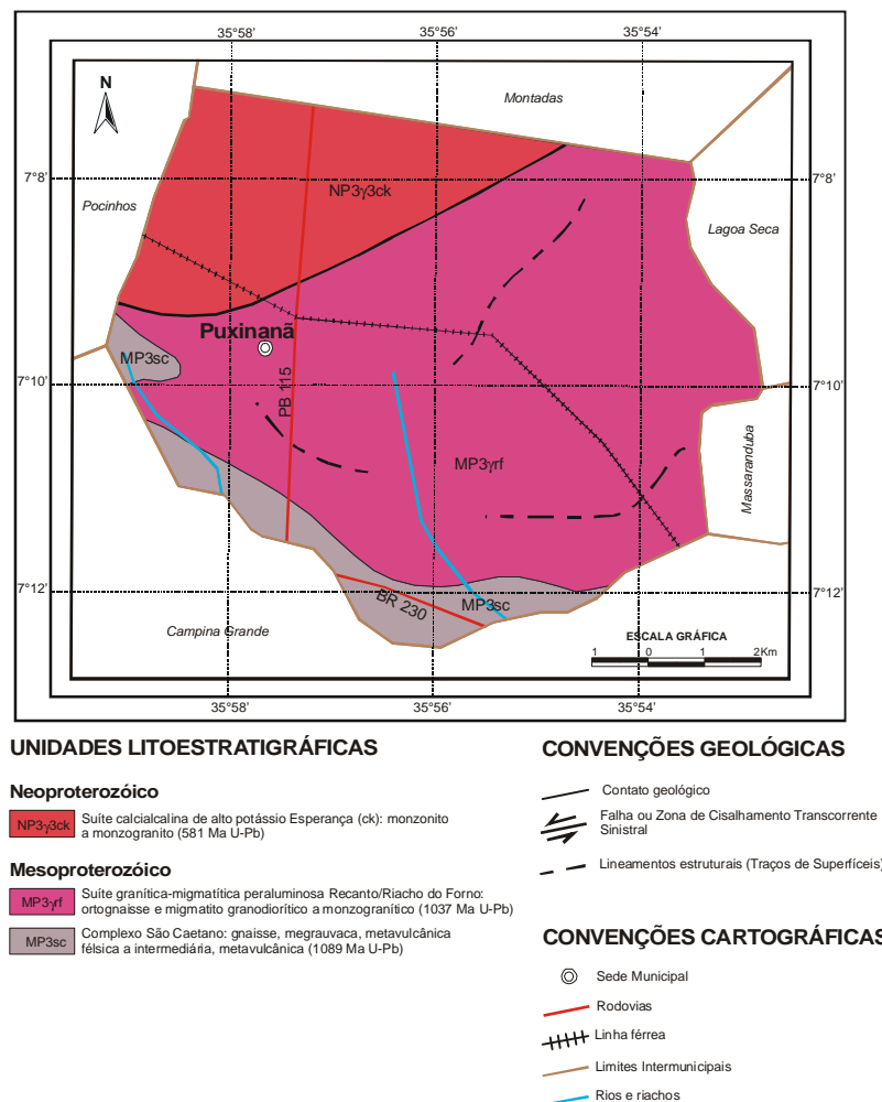
Figura 3 – Mapa Geológico
