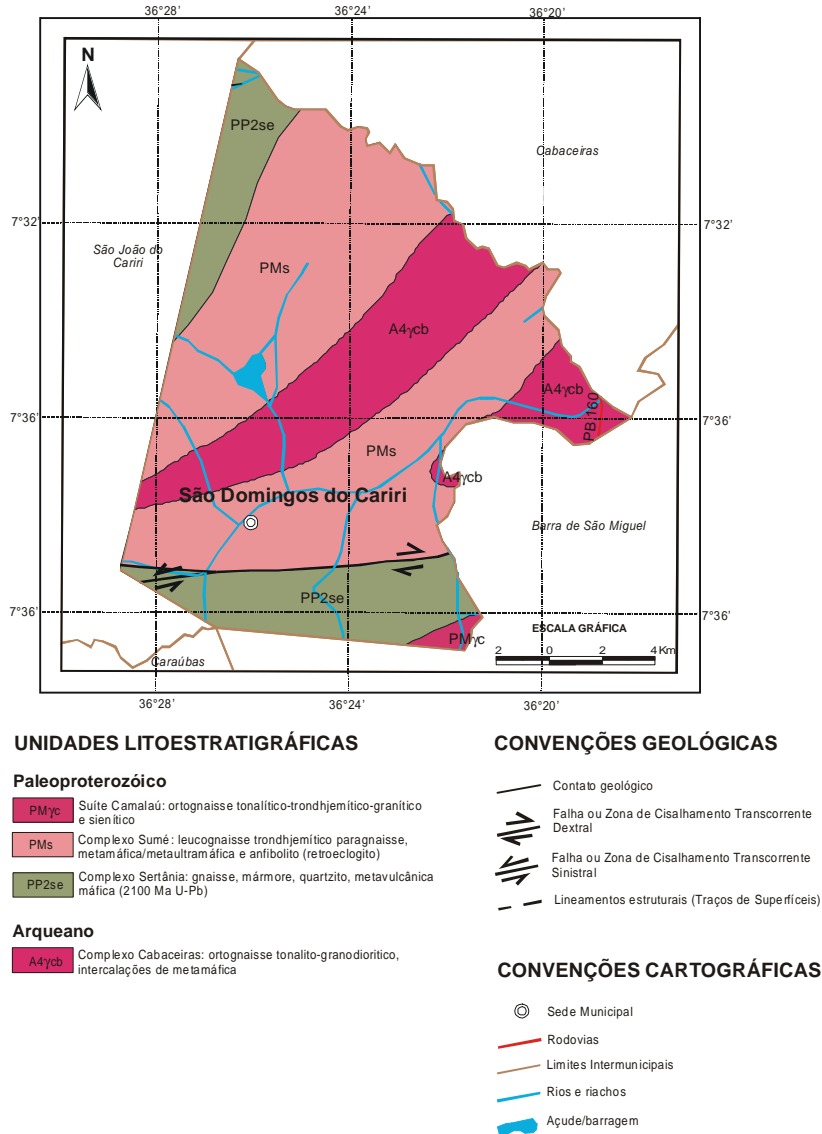
Figura 3 – Mapa Geológico
