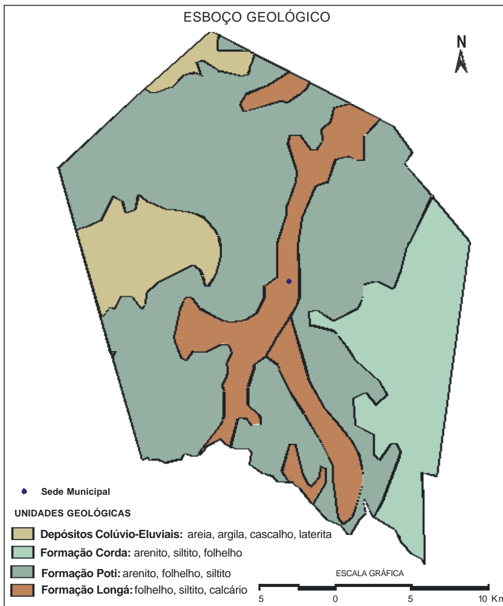
Figura 3 - Esboço geológico do município.
