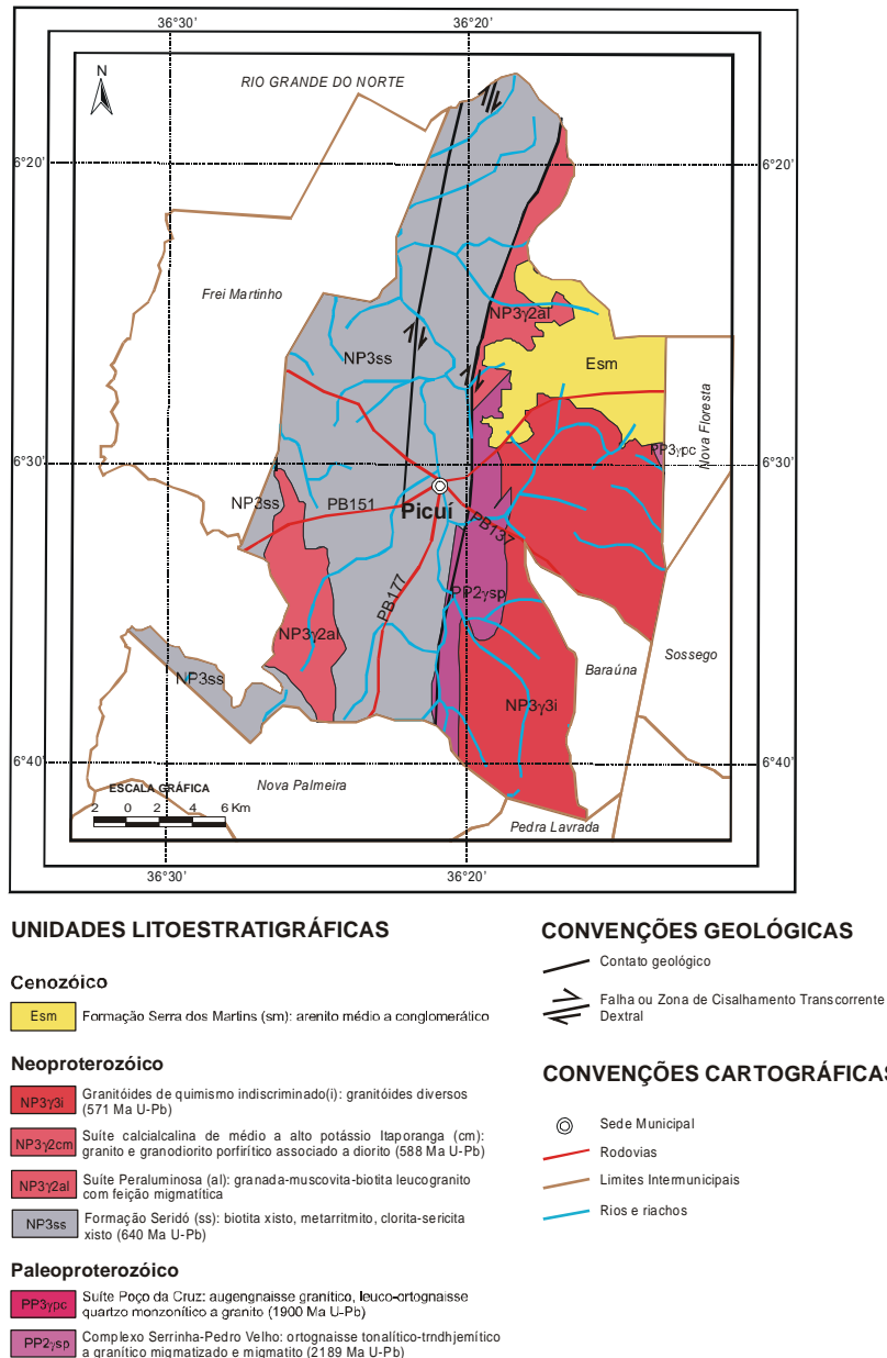
Figura 3 – Mapa Geológico
