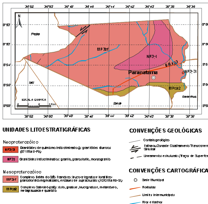
Figura 3- Mapa Geológico
