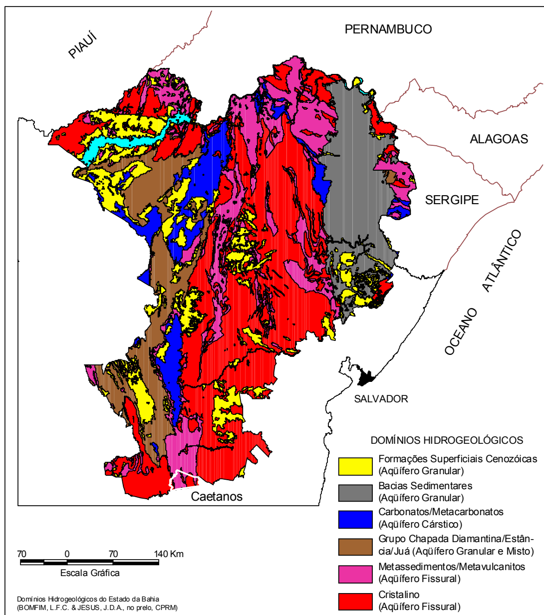
Figura 4 – Domínio hidrogeológico.
