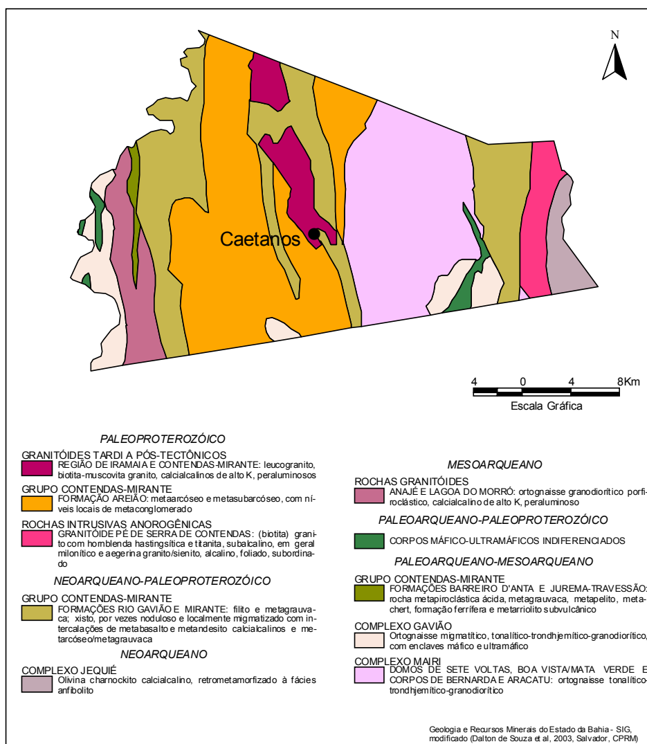
Figura 3 – Esboço geológico.
