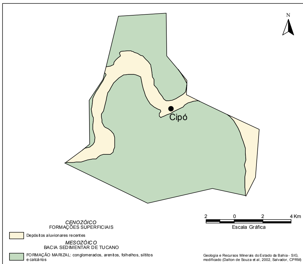
Figura 3 – Esboço geológico.
