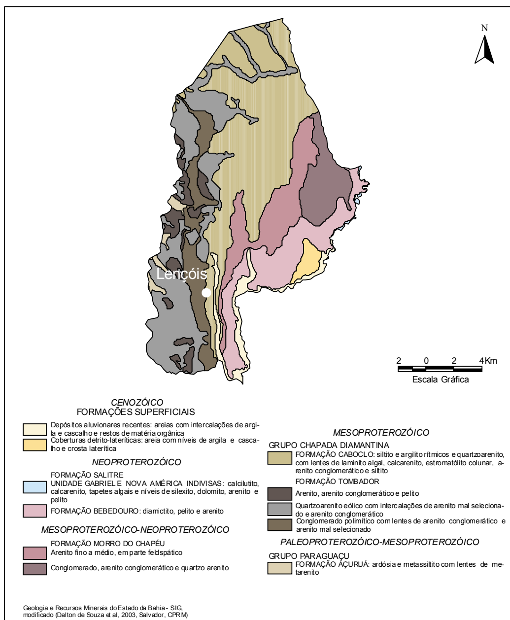
Figura 3 – Esboço geológico.
