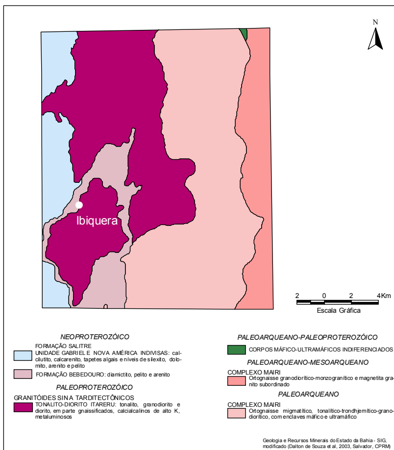
Figura 3 – Esboço geológico.
