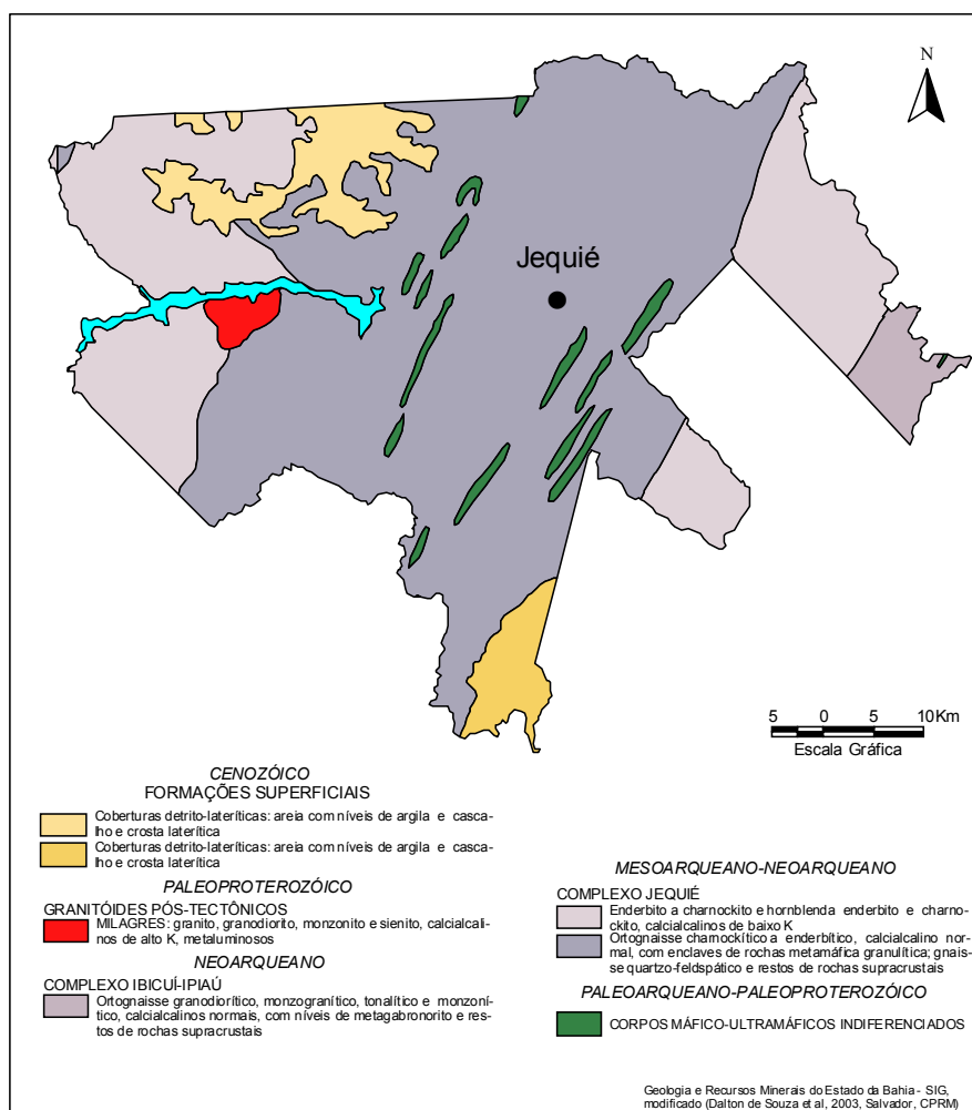
Figura 3 – Esboço geológico.
