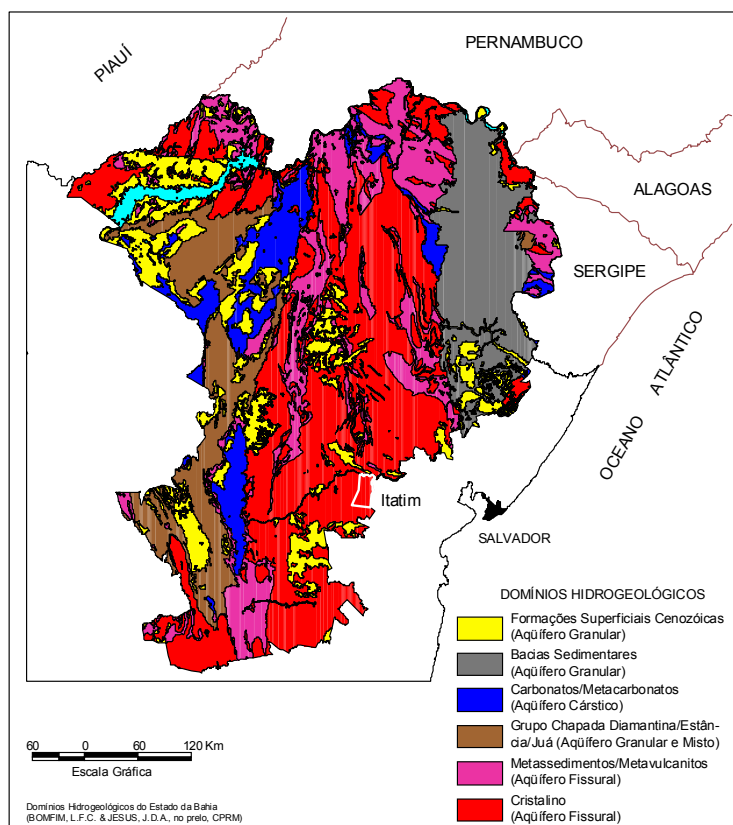
Figura 4 – Domínio hidrogeológico.
