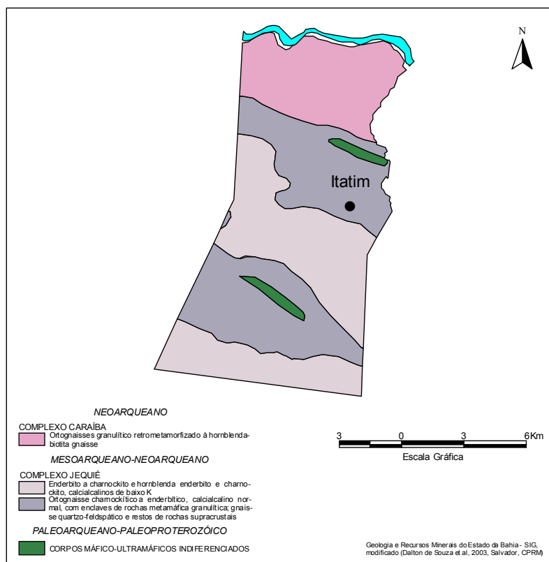
Figura 3 – Esboço geológico.
