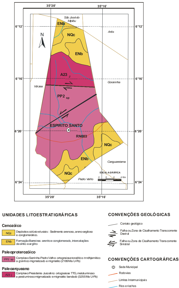
Figura 3 - Mapa Geológico
