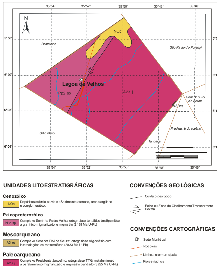
Figura 3 - Mapa Geológico
