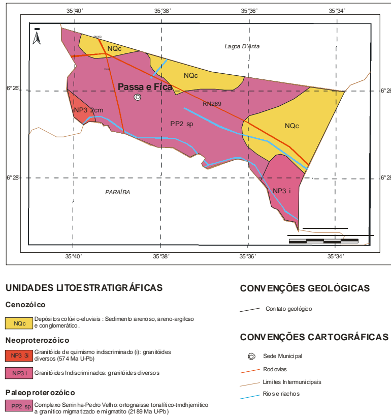
Figura 3 - Mapa Geológico
