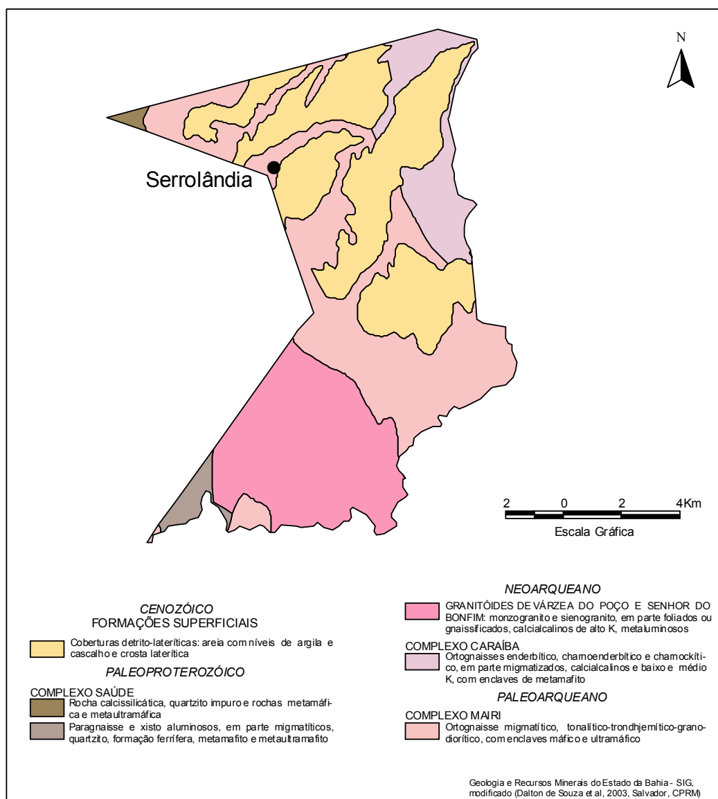
Figura 3 – Esboço geológico.
