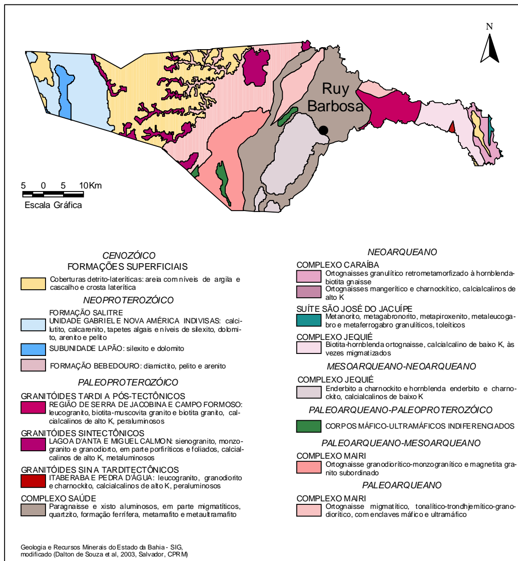
Figura 3 – Esboço geológico.
