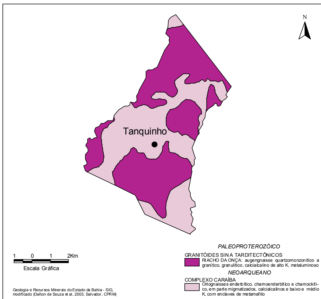
Figura 3 – Esboço geológico.
