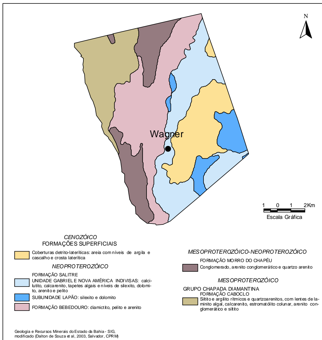
Figura 3 – Esboço geológico.
