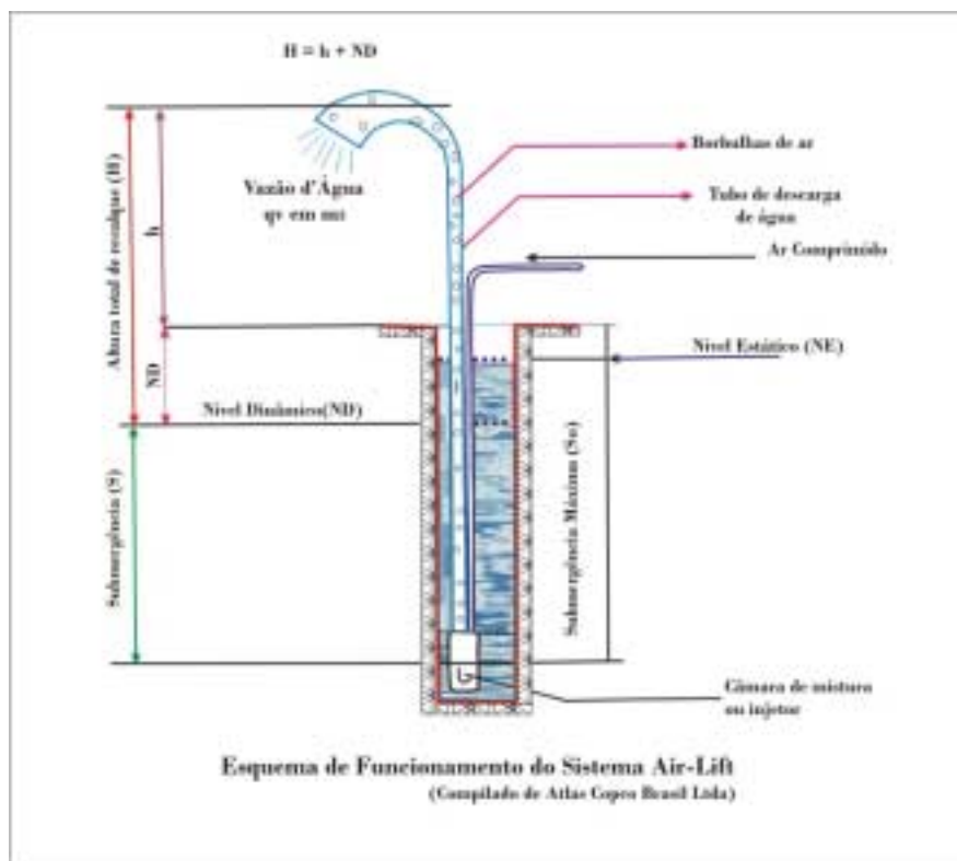
Figura 5.1 - Esquema de funcionamento do Sistema "Air Lift"
