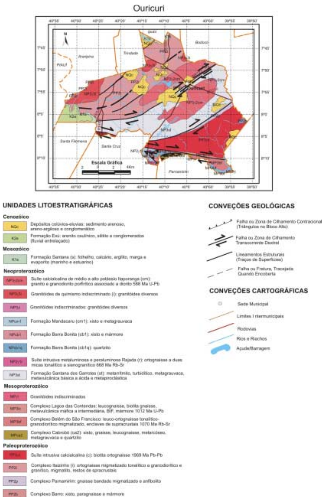
Figura 4.1 - Mapa geológico de Ouricuri - PE
