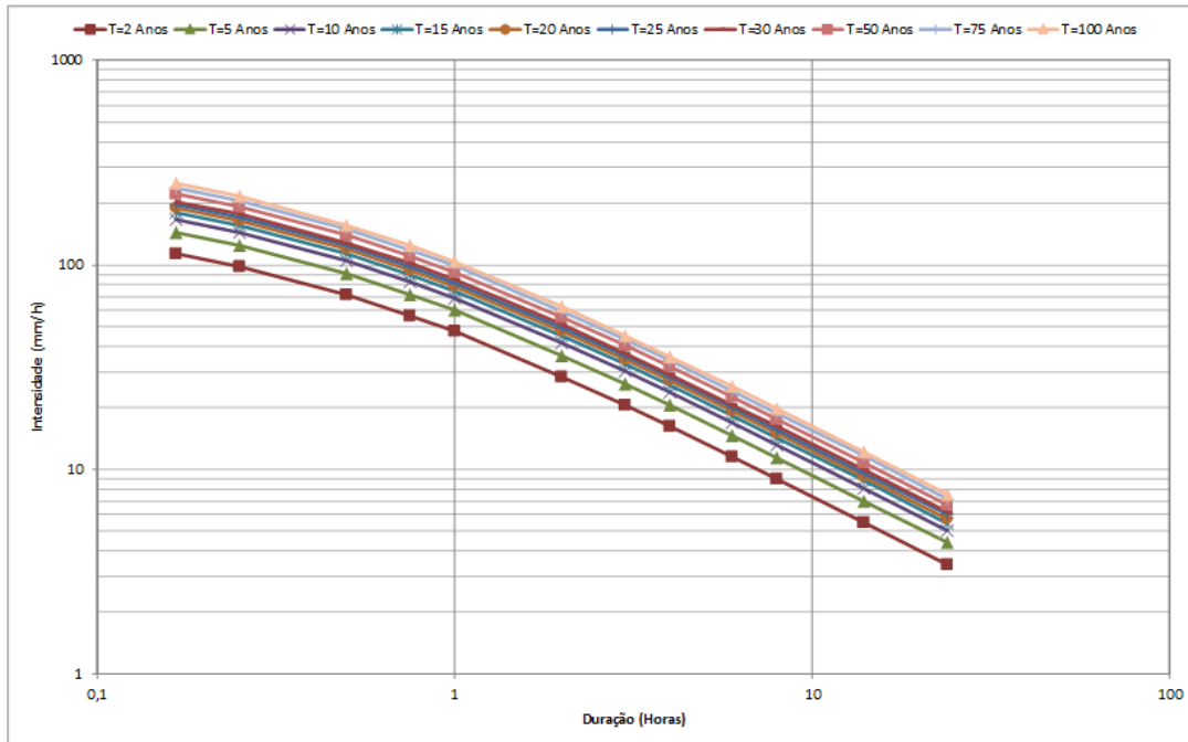
Figura 02 – Curvas intensidade-duração-freqüência
