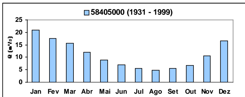
Figura 4 - Vazões médias mensais do rio Piabanha em Pedro do Rio
