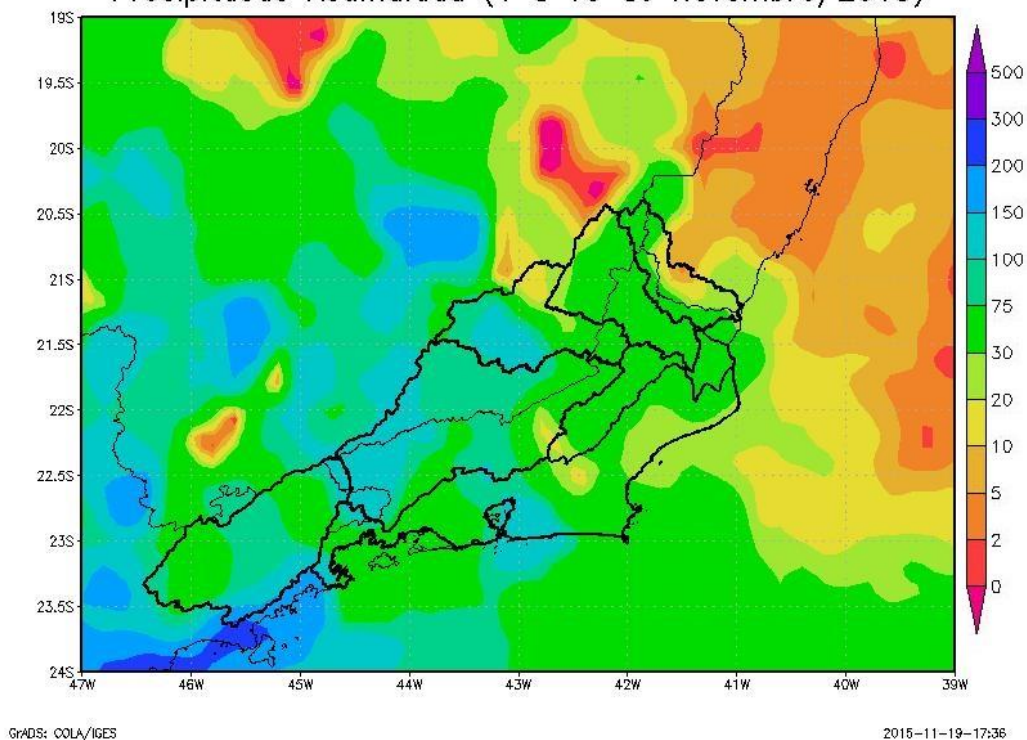
Figura 2 - Precipitação acumulada nos primeiros 15 dias de novembro de 2015.
