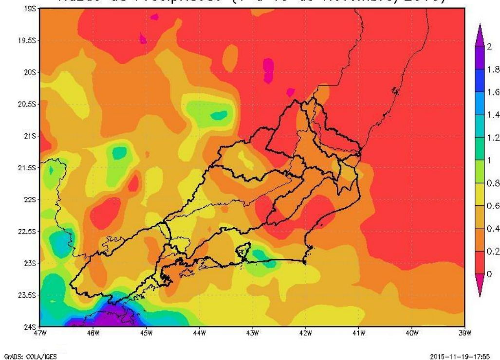
Figura 3 – Razão entre a precipitação acumulada nos primeiros 15 dias do mês de novembro de 2015 e a média histórica de novembro (1998 a 2013).
