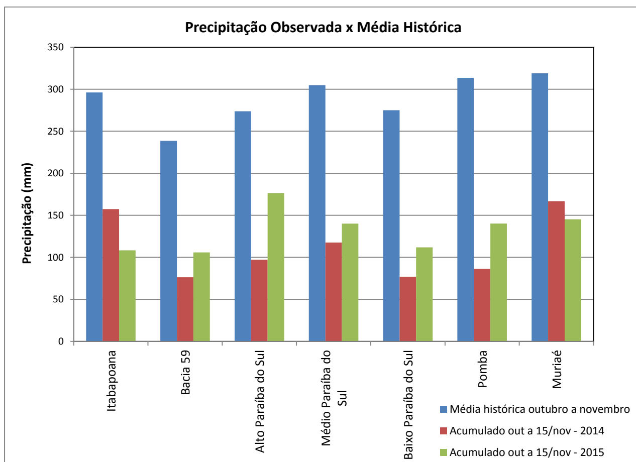
Figura 4 - Comparação entre a precipitação média histórica de outubro a novembro, a precipitação acumulada de outubro a 15 de novembro de 2014, e a precipitação acumulada de outubro a 15 de novembro de 2015 nas bacias da área de atuação da SUREG/SP.
