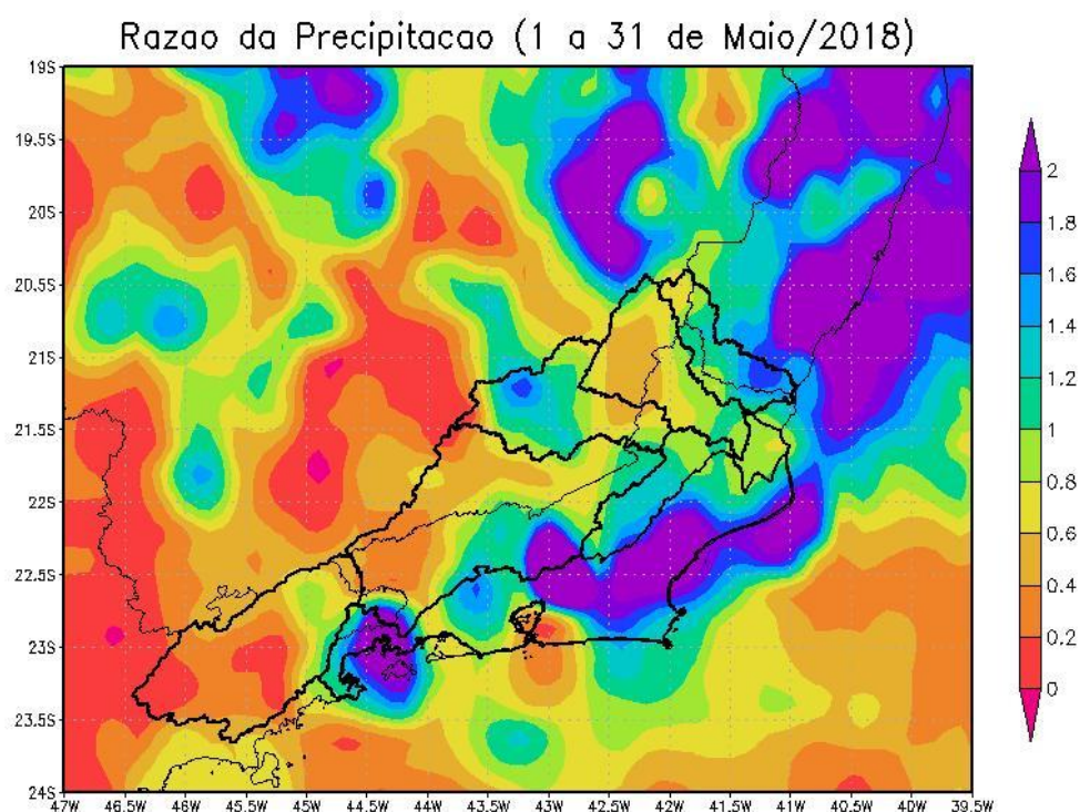
Figura 4 – Razão entre a precipitação acumulada no mês de maio de 2018 e a média histórica de maio (1998 a 2013).
