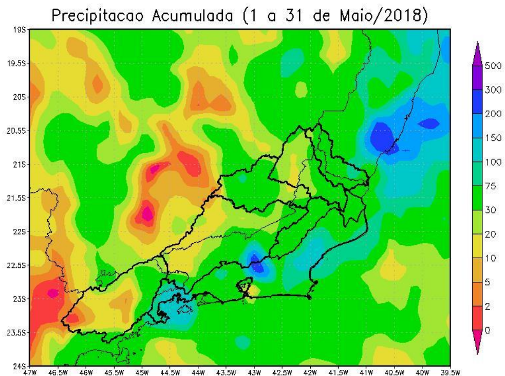
Figura 3 - Precipitação acumulada no mês de maio de 2018
