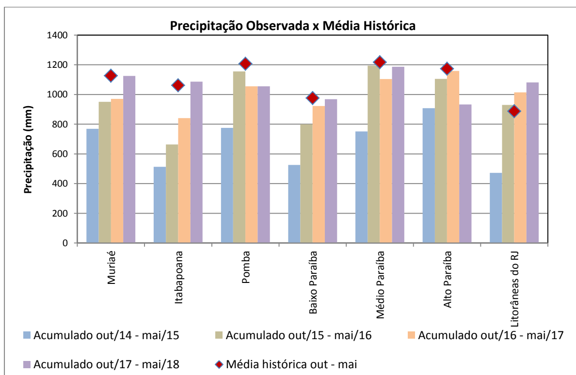
Figura 5 - Comparação entre a precipitação média histórica de outubro a maio, e a precipitação acumulada de outubro a maio de 2015, 2016, 2017 e 2018 nas bacias da área de atuação da SUREG/SP.
