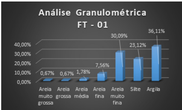
Quadro B.1: Gráfico ilustrando o resultado da análise granulométrica realizada nos solos coletados nos furos de trado.
