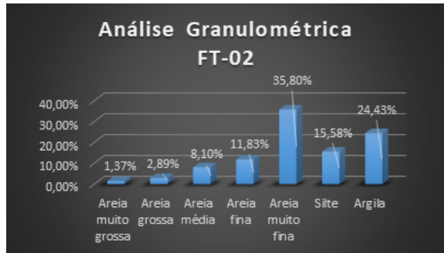
Quadro B.1: Gráfico ilustrando o resultado da análise granulométrica realizada nos solos coletados nos furos de trado.
