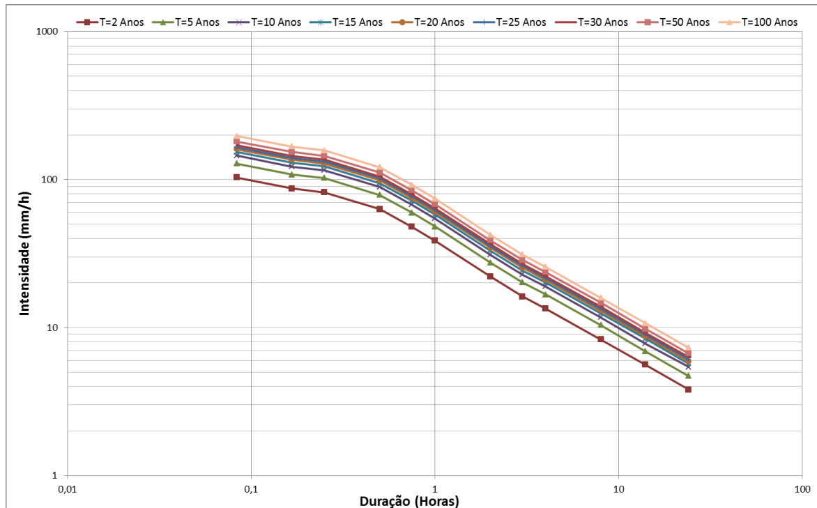
Figura 02 – Curvas intensidade-duração-frequência
