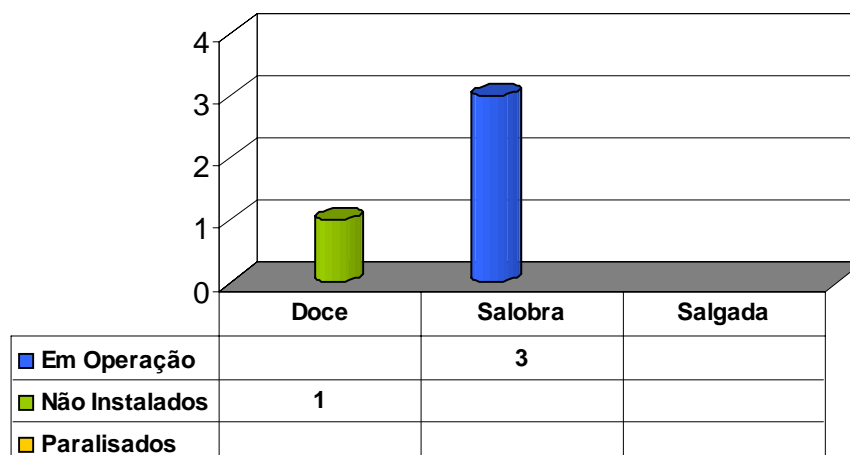
Figura 8 – Qualidade das águas subterrâneas nos aquíferos tipo granular
