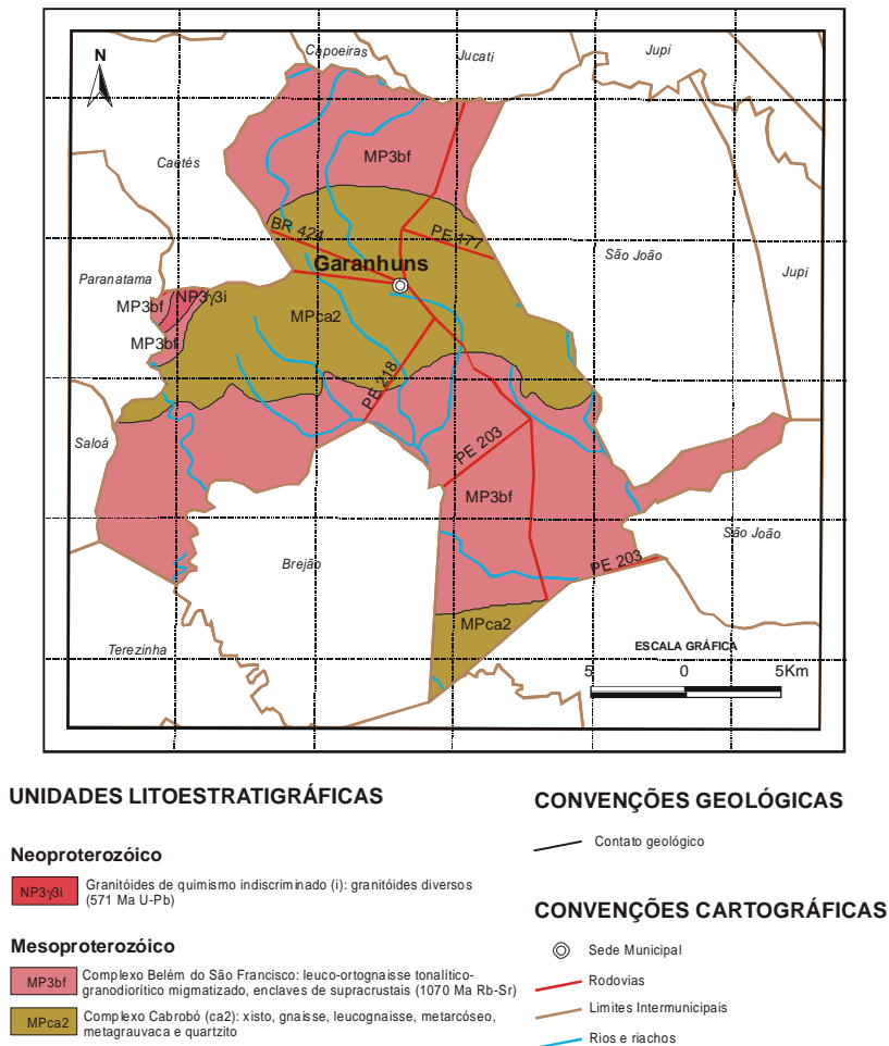
Figura 3 – Mapa Geológico
