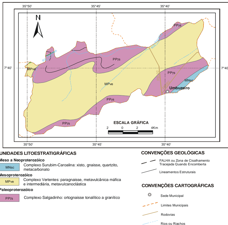
Figura 3 – Mapa Geológico
