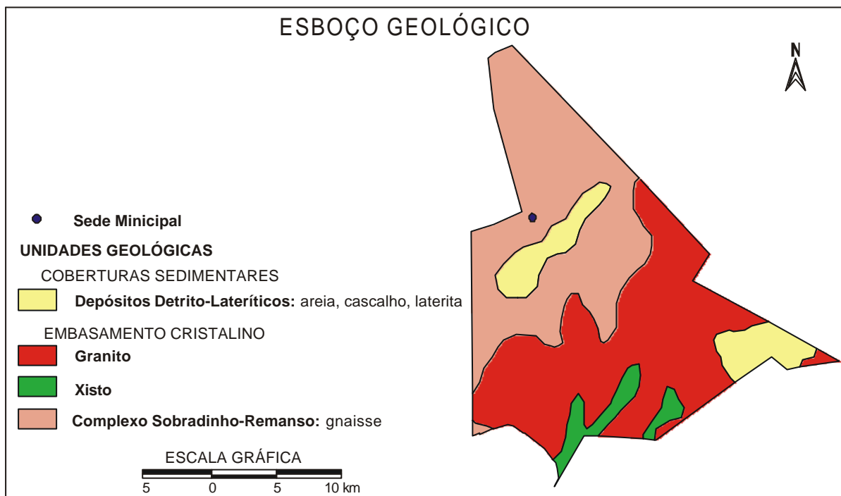
Figura 3 - Esboço geológico do município.
