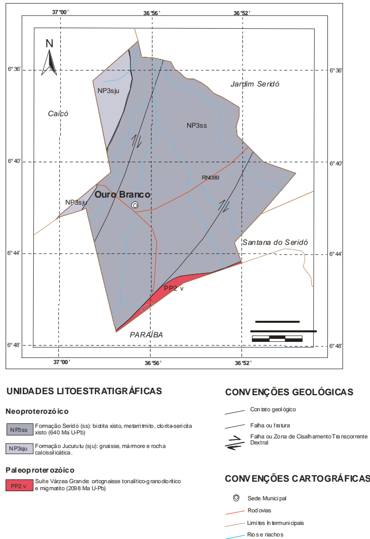
Figura 3 - Mapa Geológico
