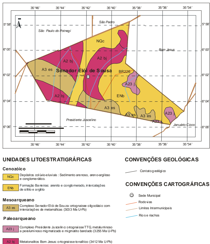
Figura 3 - Mapa Geológico
