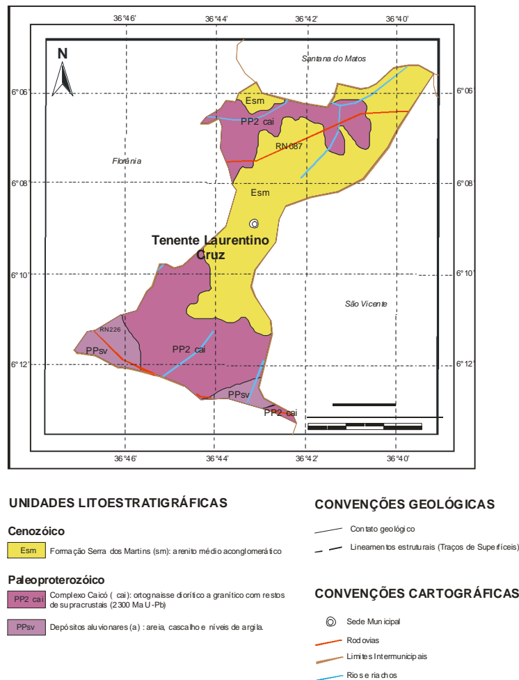
Figura 3 - Mapa Geológico
